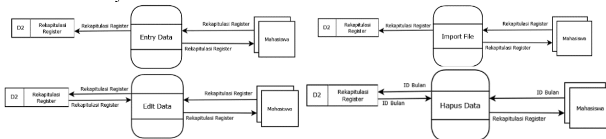
Gambar 6. Event diagram entry data, import file, edit data, dan hapus data prototipe aplikasi Grafik Barber Johnson
