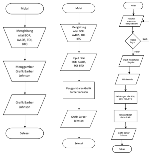
Gambar 8. Flowchart Grafik Barber Johnson manual, Microsoft Excel, dan prototipe aplikasi Grafik Barber Johnson
