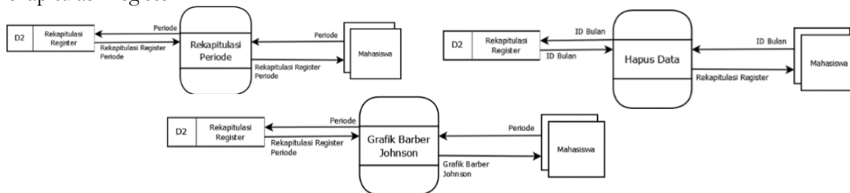
Gambar 7. Event diagram rekapitulasi register, hapus data, dan Grafik Barber Johnson prototipe aplikasi Grafik Barber Johnson
