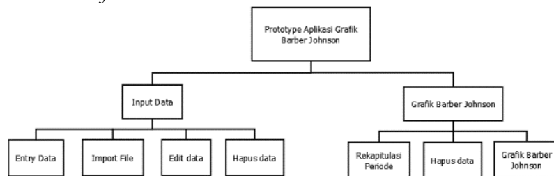
Gambar 5. Diagram dekomposisi prototipe aplikasi Grafik Barber Johnson
